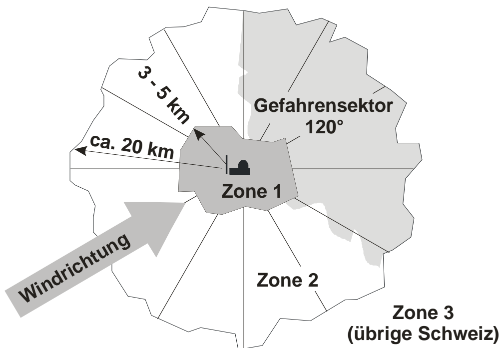
Schematische Darstellung der Gefahrensektoren in der Zone 2 um ein KKW
